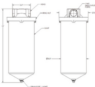
Carcaça para cartuchos filtrantes de 4" a 4,5"
