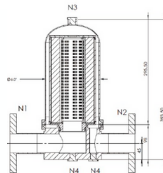
Carcaça para cartuchos filtrantes de 5,2"
